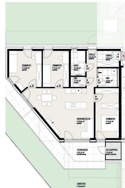
4-Zimmer-Gartenwohnung Top 13
